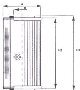
FIG. 1 INFORMAZIONI DIMENSIONALI
